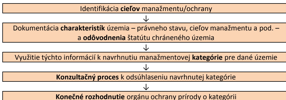
Obr. 1. Proces priradovania kategórií chráneným územiám
