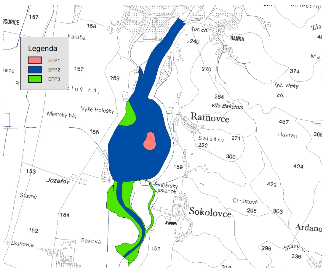
Obr. 1. Členenie CHVÚ Sĺňava na EFP
